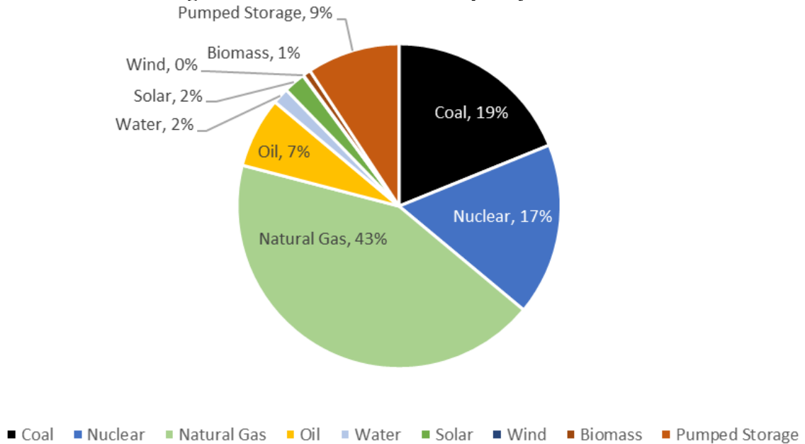
Figure 5.1.1.2 – 2022 Actual Capacity Mix
